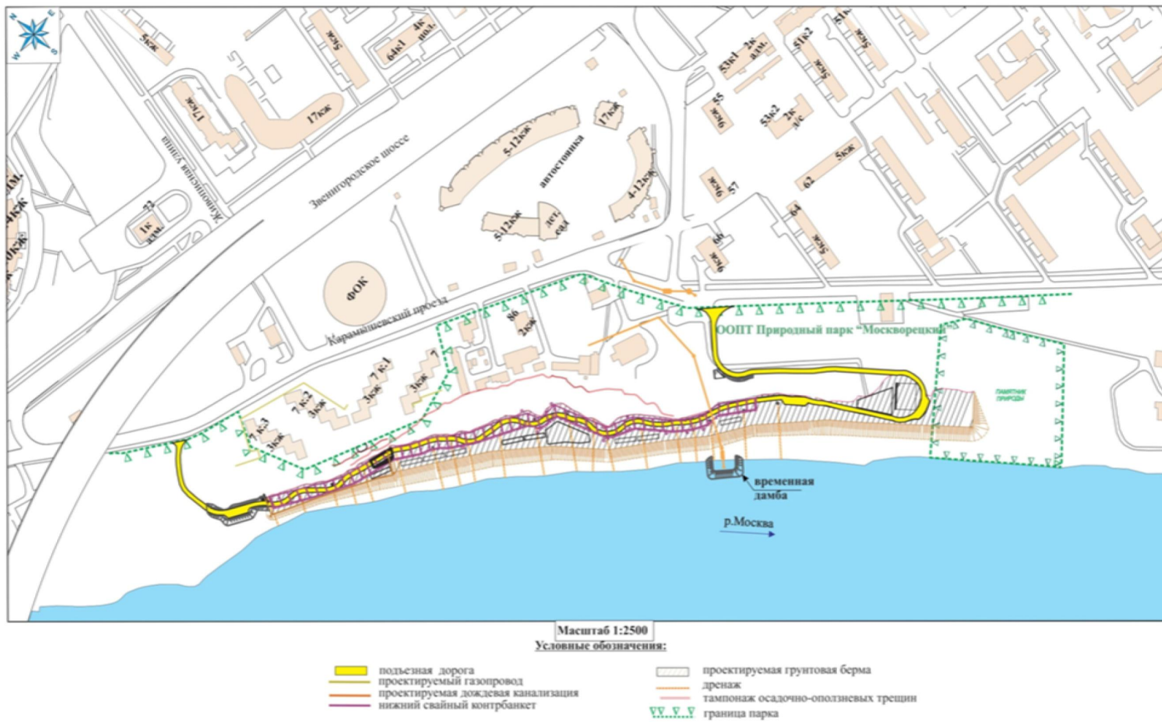
Рисунок 1.1. Схема основных проектных решений I пускового комплекса.
